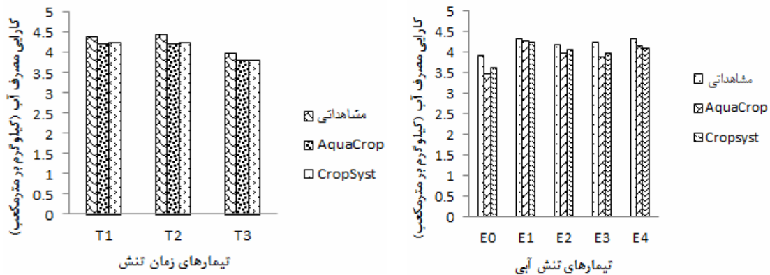
شکل ۵- مقایسه کارایی مصرف آب (کیلوگرم بر مترمکعب) شبیه‌سازی شده توسط مدل‌های AquaCrop و Cropsyst با مقادیر مشاهداتی در مقادیر مختلف تنش آبی
